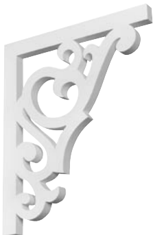
950-310 Bracket Height: 12" Width: 1" Proj.: 10"
