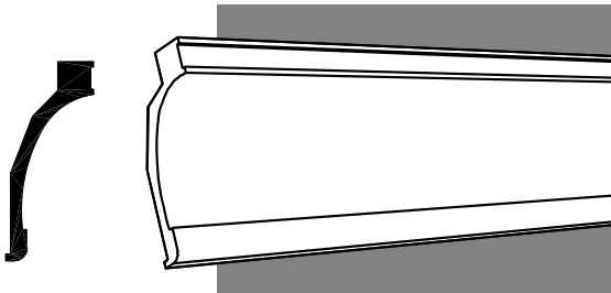
550-186-10 Moulding Ht.: 18 1/8" Length: 10' Proj.: 7 1/2"
