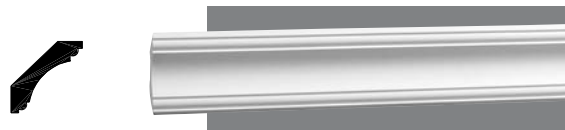
550-246-16 Moulding Ht.: 2 1/2" Length: 16' Proj.: 2 1/2"
