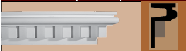
MMLD 2152B-16 Hght 2" x Proj 1" x 16'
