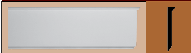
MMLD 1080-16 Hght 14-1/2" x Proj 2-1/16" x 16'
