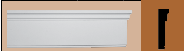
MMLD 2504-8 Hght 4-3/4" x Proj 3" x 8'
