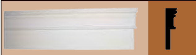
MMLD 1034-16 Hght 3-1/2" x Proj 1" x 16'
